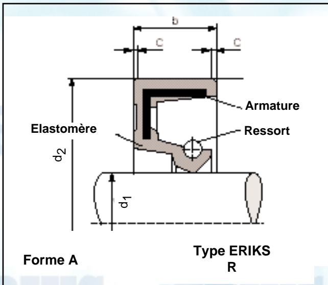
Bague d'étanchéité sans lèvres anti-poussière
