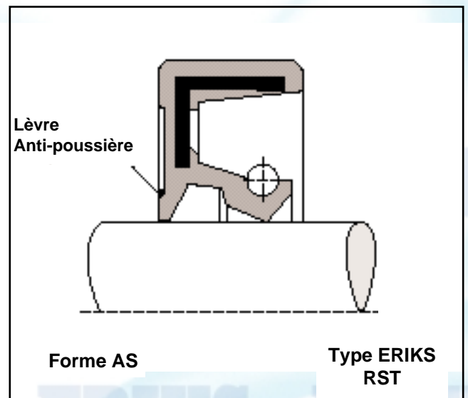
Bague d'étanchéité avec lèvres anti-poussière Les cotes sont identiques à celles de la forme A
